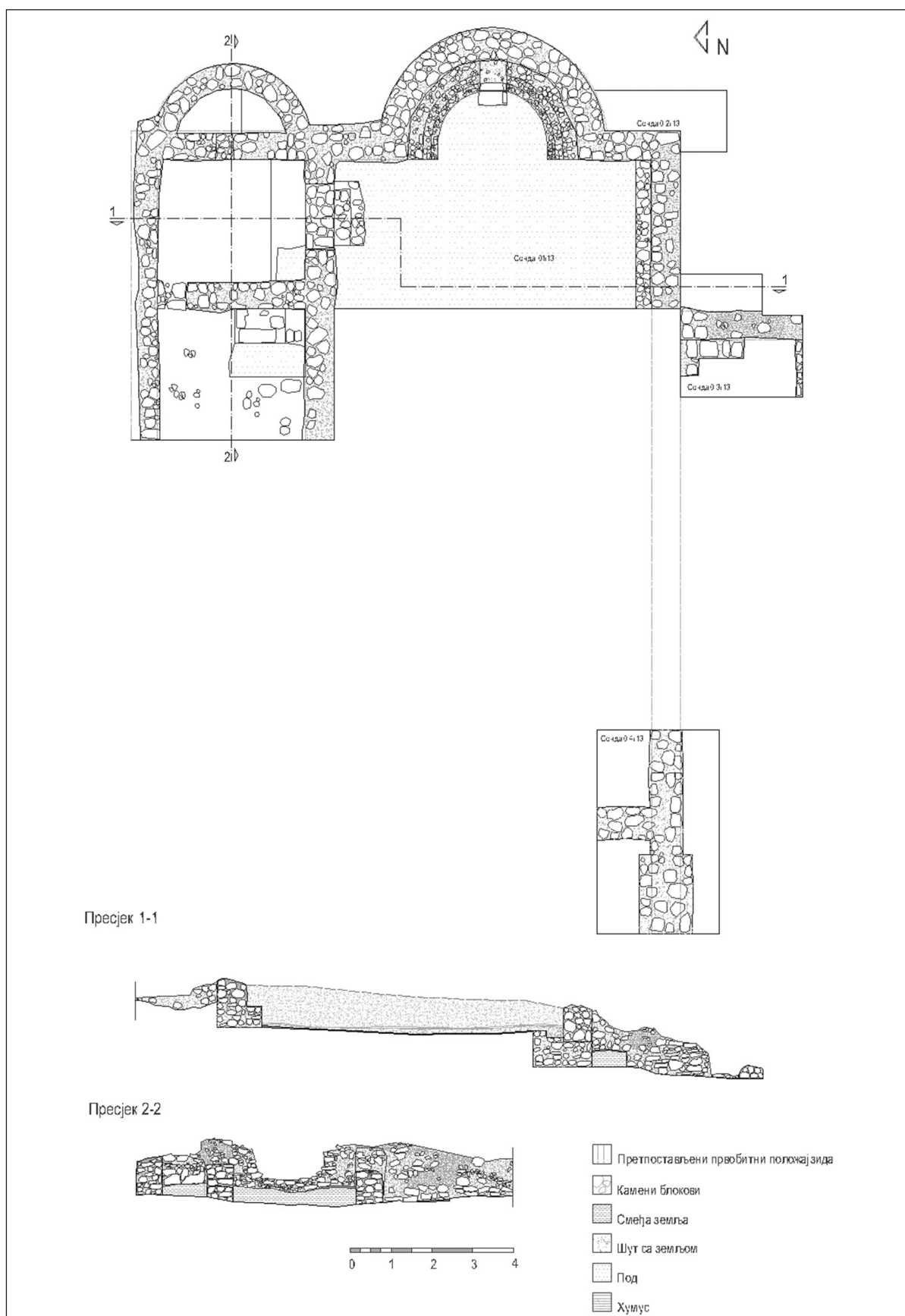
Sl. 21. Osnova i profili bazilike „B“ – sondažna istraživanja
