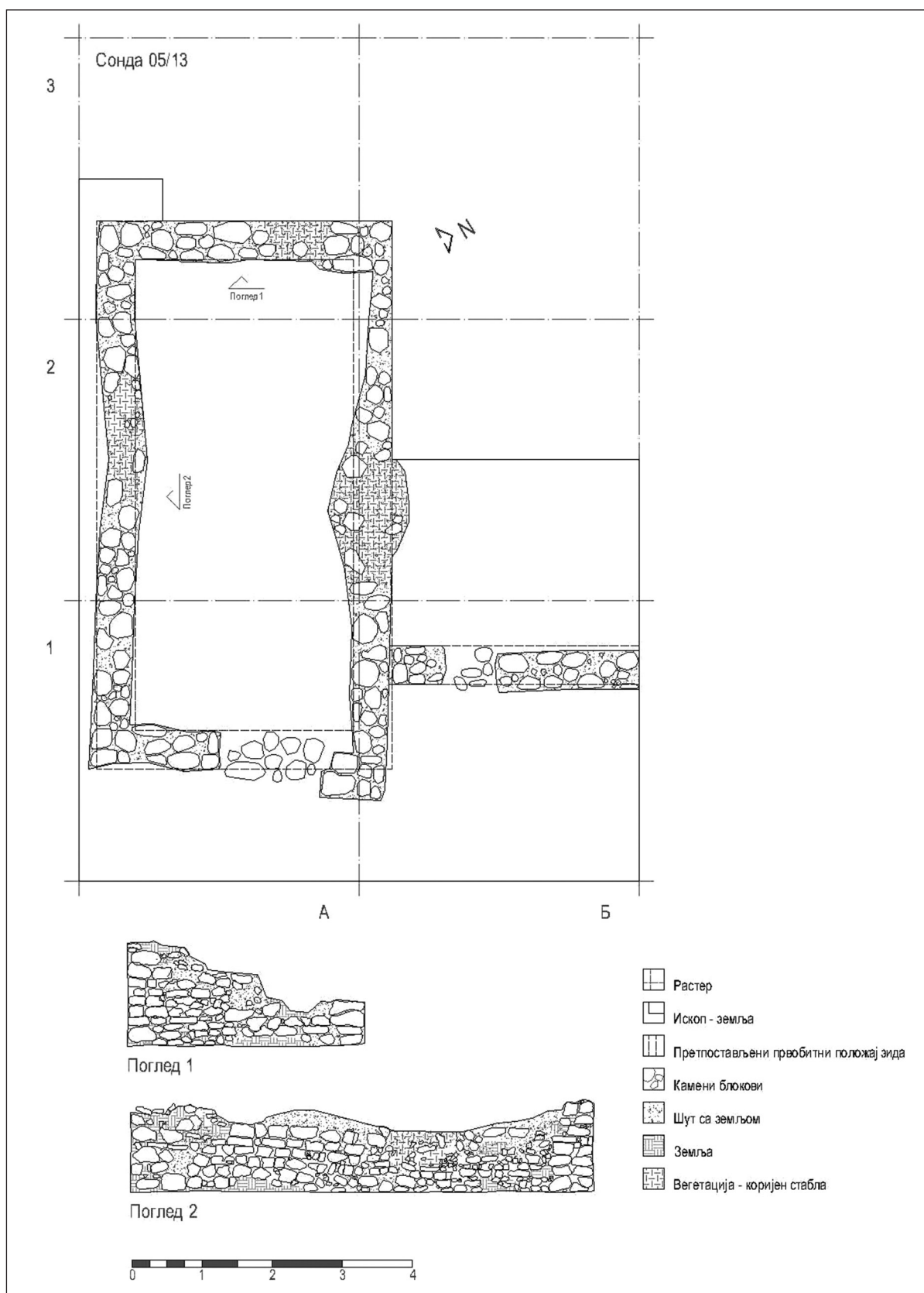
Sl. 29. Osnove i profili sondažnih istraživanja Gornjeg grada – Gradina u Bakincima
