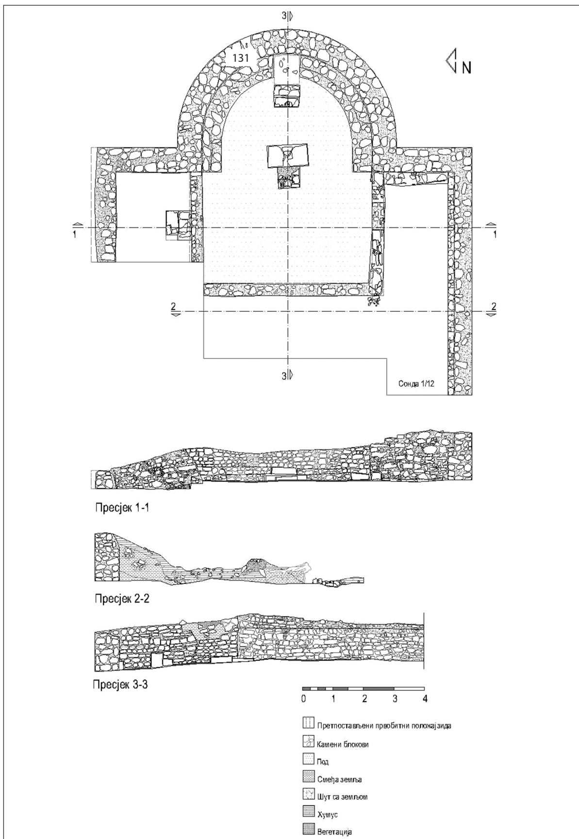
Sl. 7. Osnove i profili sondažnog istraživanja bazilike „A“ na lokalitetu Gradina u Bakincima
