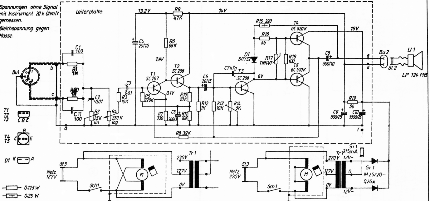
Stromlaufplan Solid 3/8
