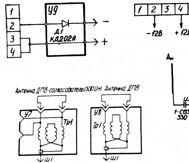
Подключения для телевизора „Шиллис 402Д-1“
