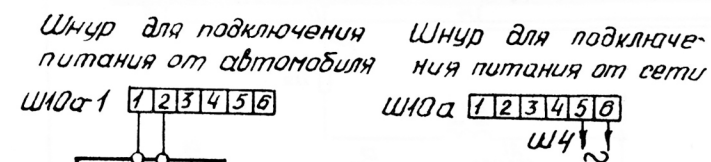
Подключения для телевизора „Шиллис 402Д-1“
